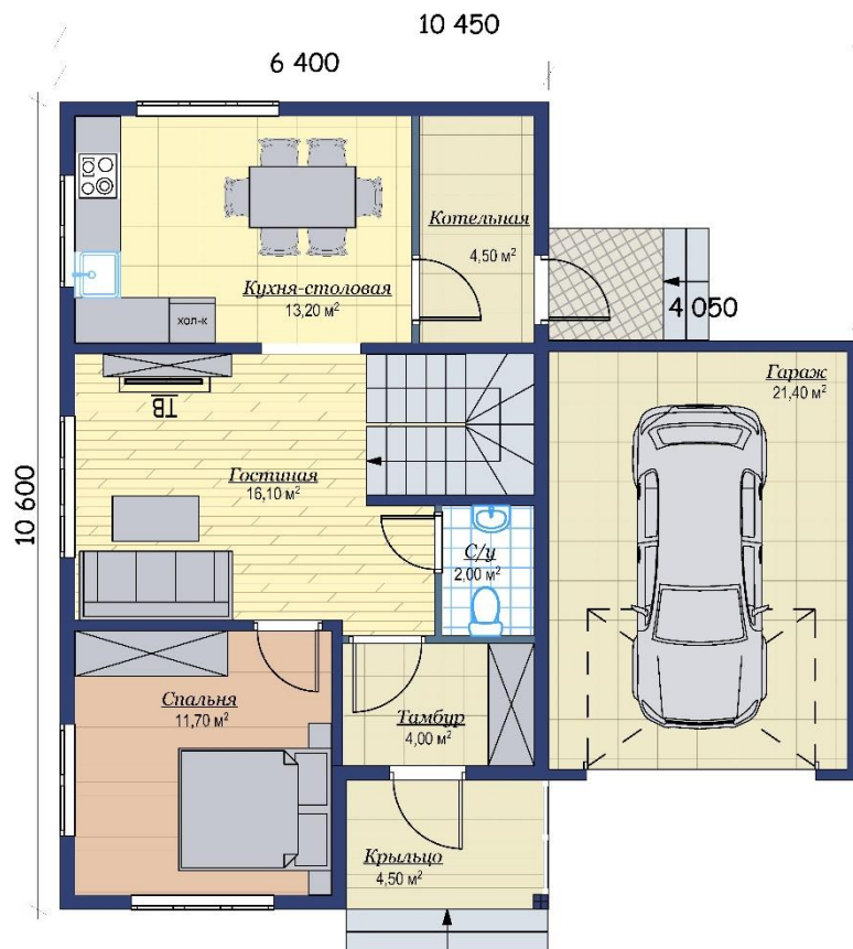
План 1-го этажа
