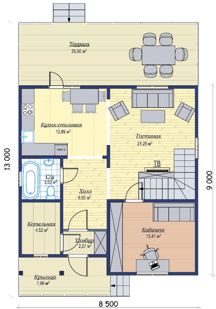
План 1-го этажа
